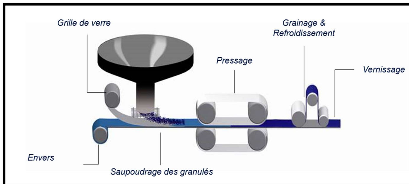
Figure 1 : Processus de Pressage
